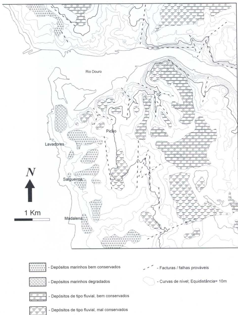
Figura 7. Esboço geomorfológico da área de Lavadores.
