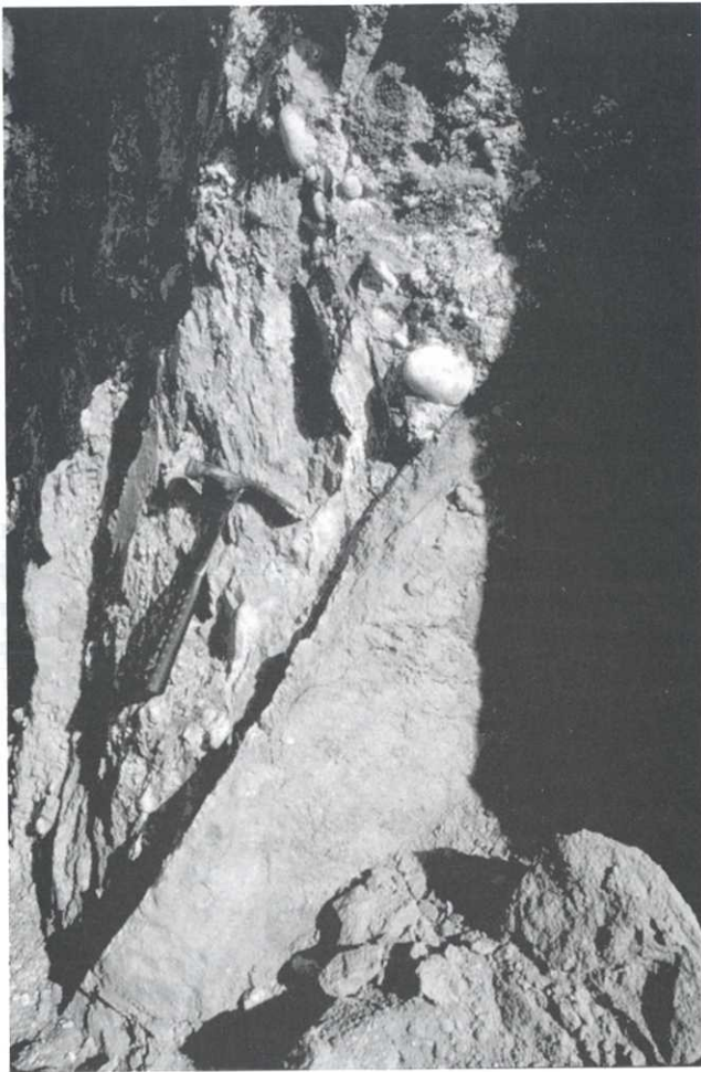
Figura 8. Falha do Juncal (Espinho). Direcção NNW-SSE; pendor 70^{\circ} W. A base do depósito é visível à esquerda. Trata-se de uma falha inversa com um rejeito aparentemente superior a 1m, já que a base do depósito, rica em elementos grosseiros, apenas aparece no bloco levantado (bloco da esquerda). No bloco abatido apenas se observa um nível fino do depósito. A base grosseira estaria subjacente, a um nível não observável.
