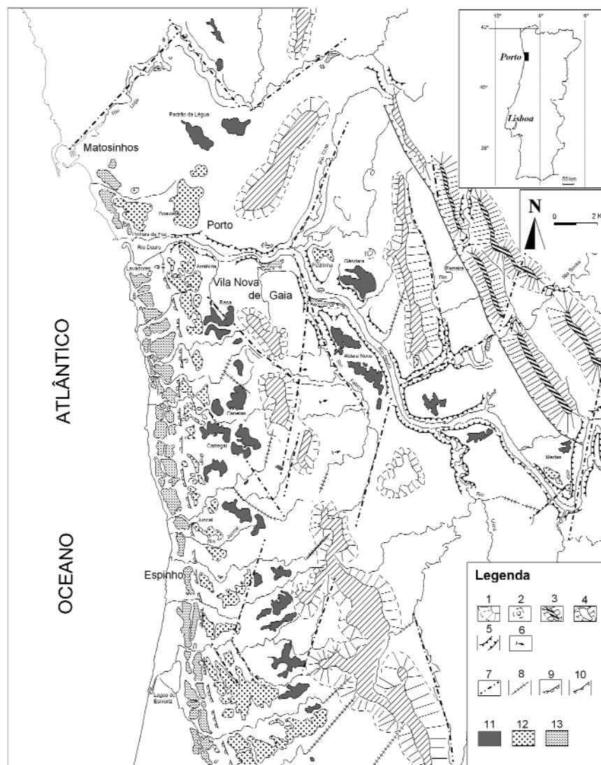
1 - Topo / base / vertente; 2 - relevo residual; 3 - crista quartzítica; 4 - relevo marginal; 5 - garganta fluvial; 6 - basculamento; 7 - falha provável; 8 - vale de fractura; 9 - escarpa de falha provável; 10 - Sulco Carbonífero Dúrico-Beirão; 11 - depósitos fluviais (fase I); 12 - depósitos fluviais (fase II); 13 - depósitos marinhos e fluviais actuais.
