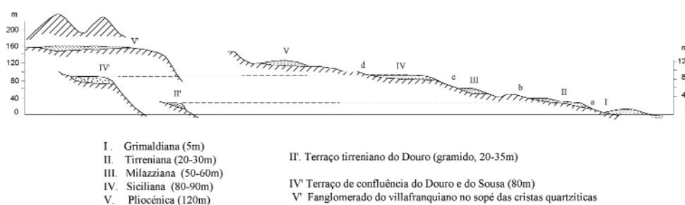
Figura 1. Corte que resume a explicação tradicional da organização do relevo nos arredores do Porto, segundo O. RIBEIRO et al. (1943).
