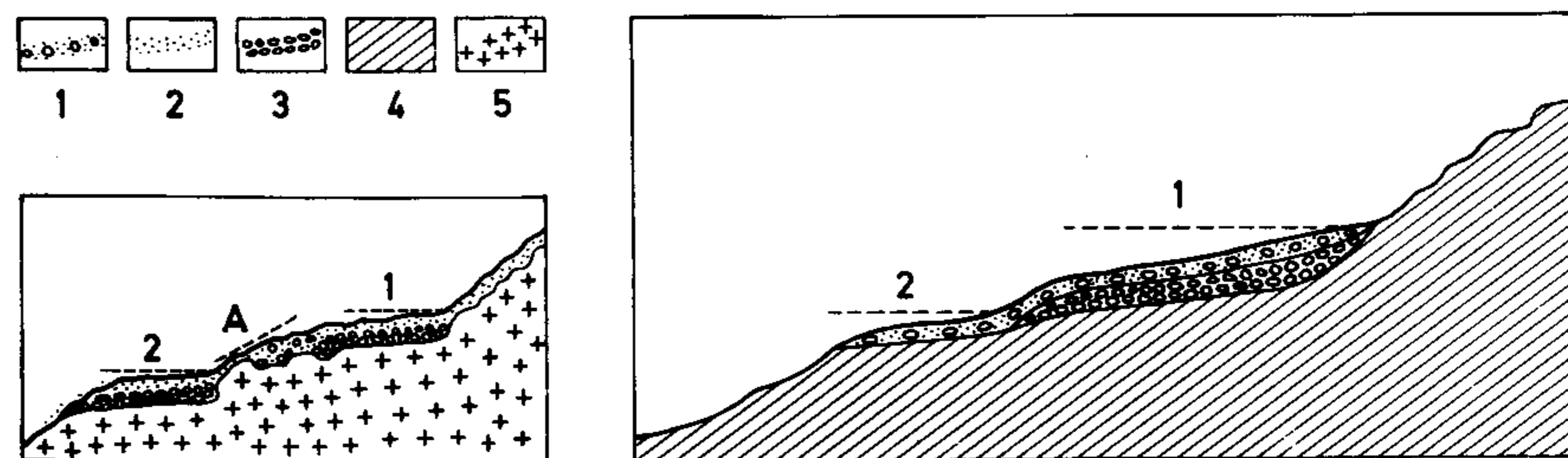
Fig. 5 — Casos de desenvolvimento de terraços. 1 - Depósitos com calhaus provenientes de terraços; 2 - coberturas mais finas; 3 - terraços; 4 - rochas de suporte de terraços; 5 - granitos.
