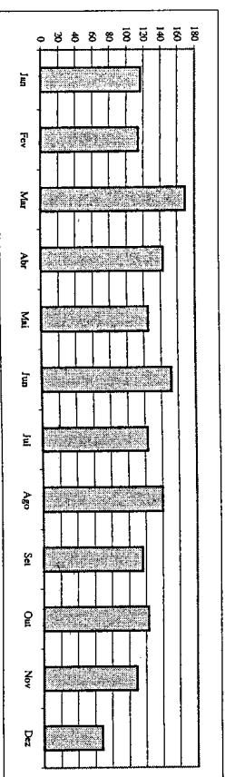
Fig. 2 - Totais mensais de tentativas de suicídio entre 1991 e 1997 registadas no Hospital de S. João (Porto).
