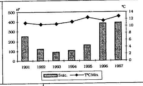
Fig.5 - Totais anuais de tentativas de suicídio e médias anuais da Temperatura Mínima
