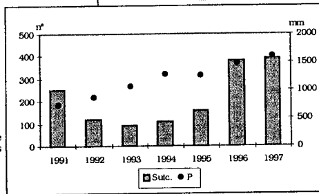
Fig.7 - Totais anuais de tentativas de suicídio e totais anuais de Precipitação
