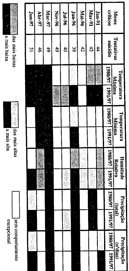
Fig. 10 – Características climatológicas excepcionais dos "meses críticos" relativamente aos mesmos meses de 1980 a 1997 e de 1991 a 1997.
