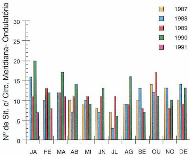
Fig. 64 – Número de situações com circulação meridiana – corrente ondulatória (entre 1 de Abril de 1987 e 31 de Março de 1991)
