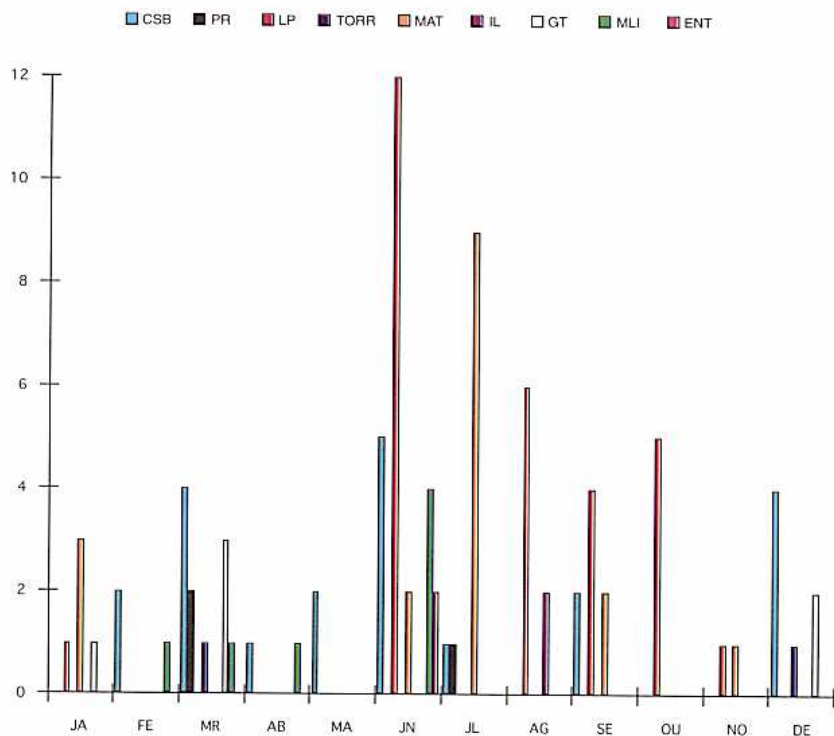
Fig. 92 – Número de dias com acidez forte acima dos 200 µg/m 3 .
