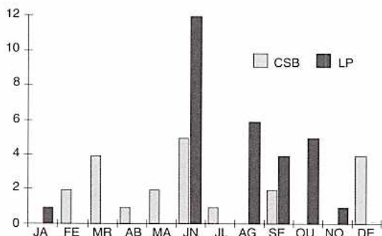
Fig. 94 – Número de dias com \text{SO}_2 acima de 200 \mu\text{g}/\text{m}^3 nos postos localizados na Casa de Saúde da Boavistá e em Leça da Palmeira (excerto da figura 92).
