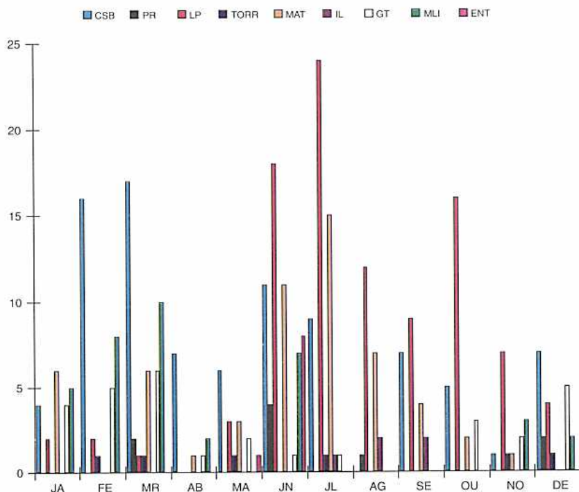
Fig. 91 – Número de dias com acidez forte acima dos 150 µg/m³.
