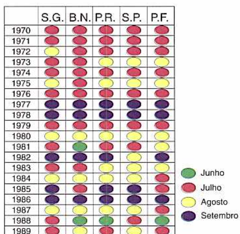
Fig. 50 – Temperatura média mensal mínima mais elevada do ano
