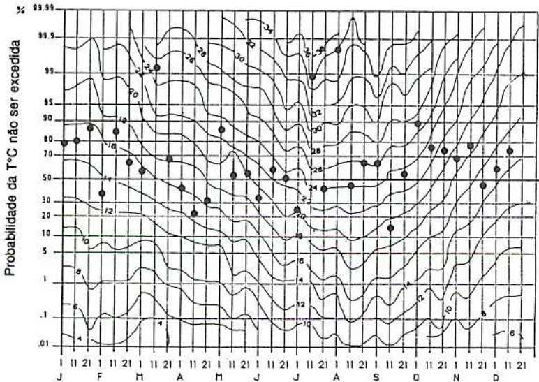
Fig. 59 – Valor de temperatura registado no Porto-Serra do Pilar nos dias 1, 11 e 21 de cada mês do ano de 1989.
