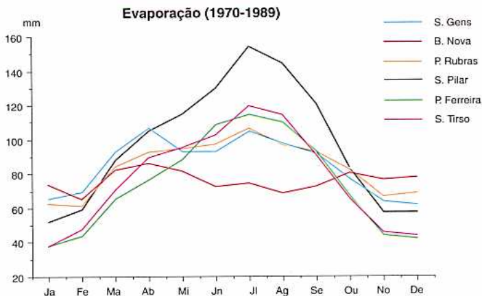
Fig. 46 – Média mensal da evaporação total (1970-1989).
