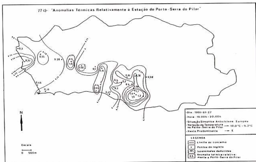
Fig. 77 c) – "Anomalias térmicas relativamente à estação do Porto-Serra do Pilar"
