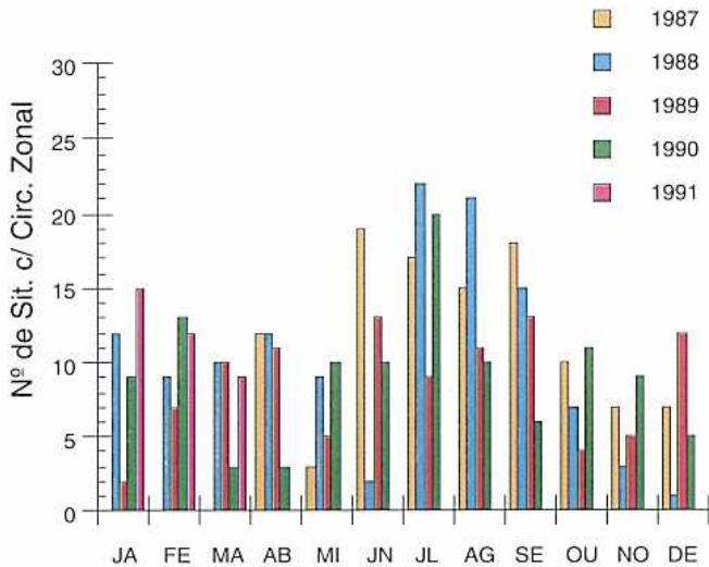
Fig. 63 – Número de situações com circulação zonal (entre 1 de Abril de 1987 e 31 de Março de 1991)
