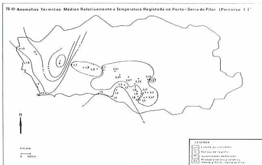
Fig. 76 a) – “Anomalias térmicas médias relativamente à temperatura registada no Porto-Serra do Pilar (Percurso 1.1)”
