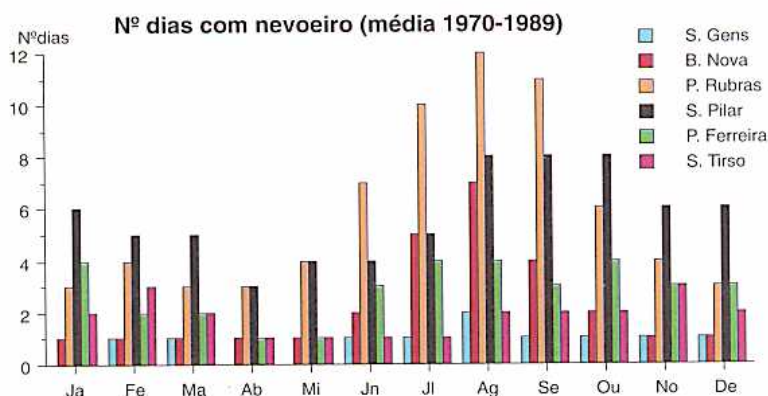
Fig. 45 – Número de dias com nevoeiro (1970-1989).
