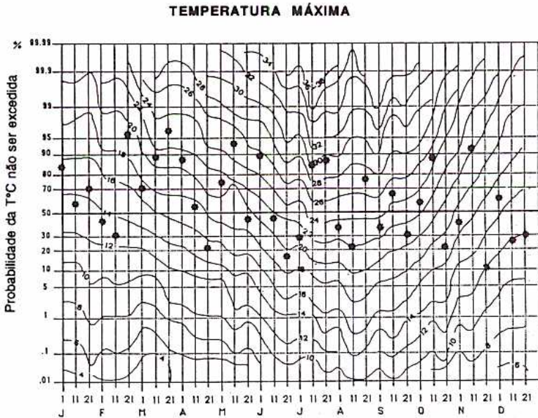
Fig. 60 – Valor de temperatura registado no Porto-Serra do Pilar nos dias 1, 11 e 21 de cada mês do ano de 1990. (o calendário de probabilidades onde foram inscritos os respectivos valores de tempera-
