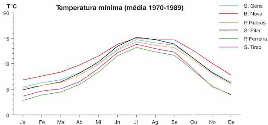
Fig. 35 a) – Temperatura média mensal mínima (1970-1989).
