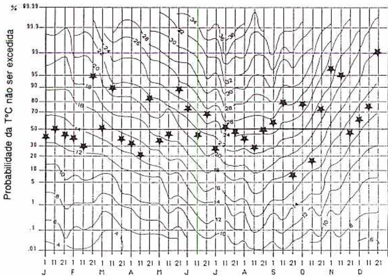
Fig. 58 – Valor de temperatura registado no Porto-Serra do Pilar nos dias 1, 11 e 21 de cada mês do ano de 1988. (o calendário de probabilidades onde foram inscritos os respectivos valores de tempera-
