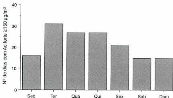
Fig. 97 – Número de dias com acidez forte \geq 150 \mu\text{g}/\text{m}^3 , em pelo menos um posto da rede de medição da qualidade do ar da DGQA-Porto, segundo o dia da semana (da 1/6/87 a 31/3/01)
