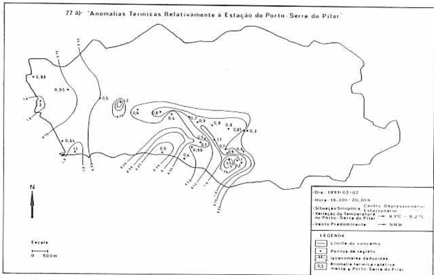
Fig. 77 a) – "Anomalias térmicas relativamente à estação do Porto-Serra do Pilar"
