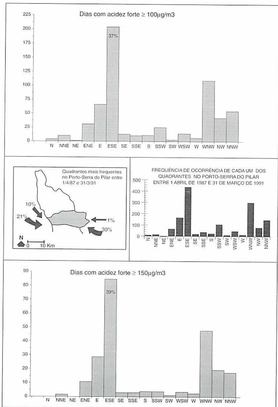
Fig. 95 – Rumo predominante do vento na estação de Porto-Serra do Pilar nos dias em que pelo menos um posto da rede da DGQA-Porto registou \text{SO}_2 \geq 100 \mu\text{g}/\text{m}^3 e \text{SO}_2 \geq 150 \mu\text{g}/\text{m}^3 .
