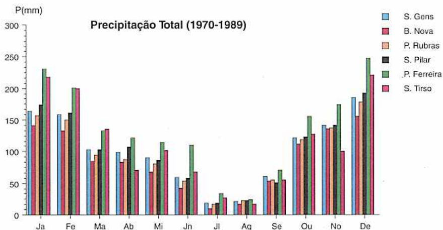
Fig. 38 – Precipitação total mensal (1970-1989).
