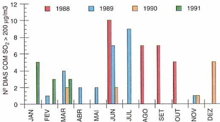
Fig. 96 – Número de dias em que o \text{SO}_2 ultrapassou 200 \mu\text{g}/\text{m}^3 em pelo menos um dos postos (ver Quadro LXIV).
