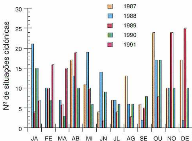
Fig. 62 – Número de situações depressionárias (entre 1 de Abril de 1987 e 31 de Março de 1991).
