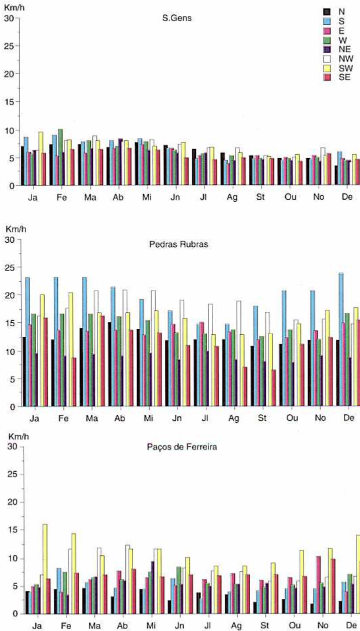
Fig. 49 – Velocidade média mensal do vento (1970-89).
