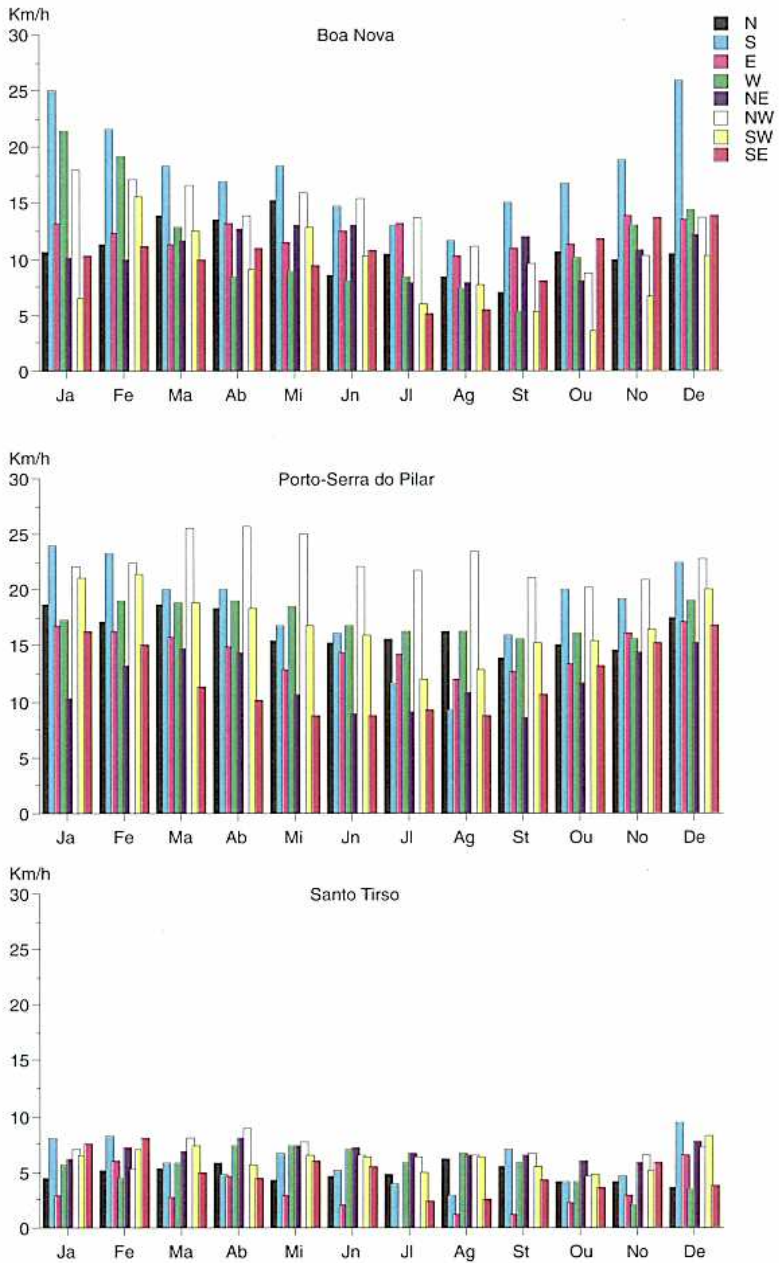
Fig. 49 (Cont.) – Velocidade média mensal do vento (1970-89).
