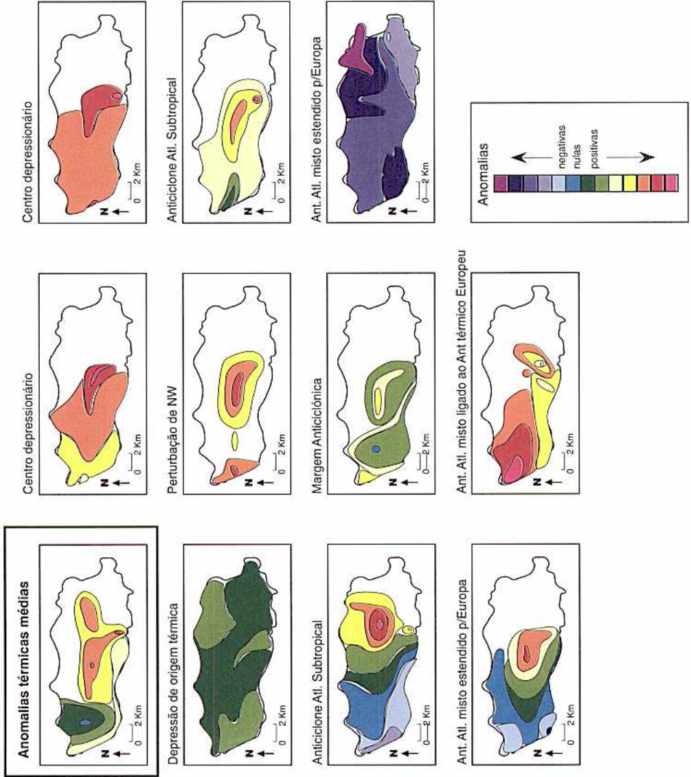
Fig. 79 – Representação esquemática das formas e intensidades da “ilha de calor” portuense sob a acção de diversas situações sinóticas.
