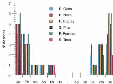
Fig. 40 – Mês mais pluvioso em cada um dos 20 anos estudados (1970-89).
